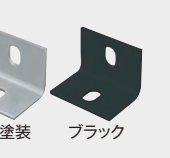
■ルーバー材固定用 ステン製Lアングル (長穴2個付) 50×50×70mm t=4mm ※無塗装、ブラックの2色から選べます
