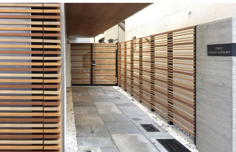
部材 20×20、20×40 アクティオーク、ジャラ、ナチュラルウッド ▶P.28
