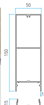
Größe in mm 50x150xL3650 t: 1.5 mm
