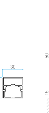
Größe in mm 30x30xL3650 t:1.0mm
