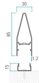
Größe in mm 30x85xL4000 Katana t: 1.2 mm
