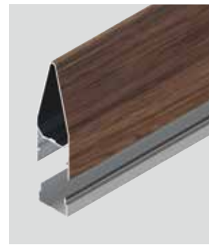
Größe in mm 30x85xL4000 Katana t: 1.2 mm
