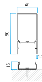
Größe in mm 40x80xL4000 t: 1.2 mm
