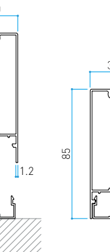
Größe in mm 30x85xL4000 t:1.2mm
