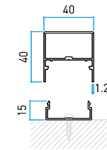
Größe in mm 40x40xL4000 t: 1.2 mm
