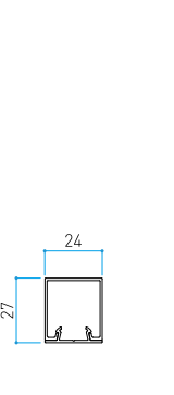
Größe in mm 24x27xL3650 t:1.0mm
