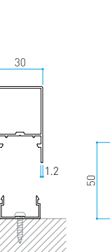
Größe in mm 30x50xL4000 t:1.2mm
