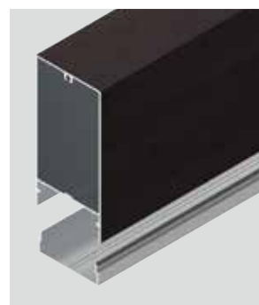
Größe in mm 50x100xL3650 t: 1.3 mm
