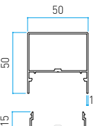
Größe in mm 50x50xL3650 t: 1.2 mm
