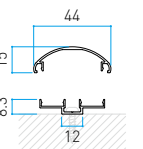
Größe in mm 44x15xL3560 t: 1.0 mm
