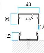
Größe in mm 40x20xL4000 t: 1.0 mm
