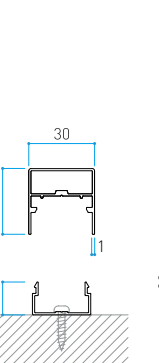
Größe in mm 30x30xL3650 t:1.0mm
