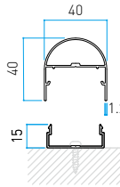
Größe in mm 40x40xL4000 t: 1.2 mm
