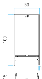
Größe in mm 50x100xL3650 t: 1.3 mm
