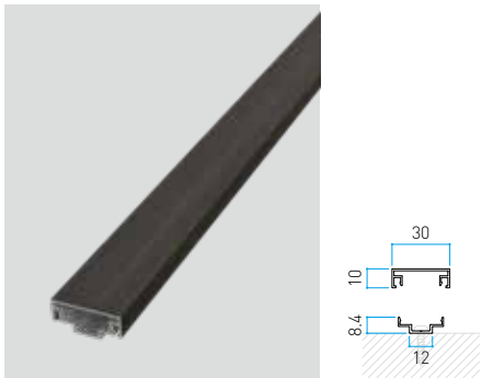
Size in mm 30x13xL3650 t: 1.0 mm
