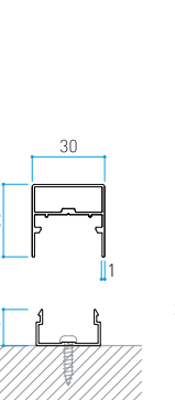
Size in mm 30x30xL3650 t:1.0mm
