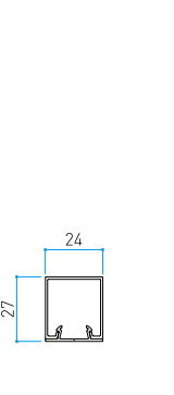
Size in mm 24x27xL3650 t:1.0mm
