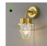
HBF-D30B W120xD185xH295mm 4.0W 2700K 224lm
