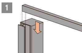
Hフレーム付きアルミ柱にアルミ脚縁を落とし込み、Hフレームの下部で固定します。
