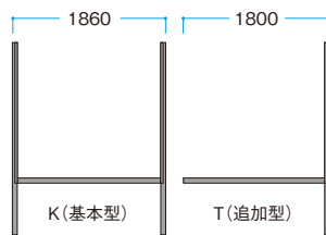
Hフレーム付きアルミ柱にアルミ脚縁を落とし込み、Hフレームの下部で固定します。
