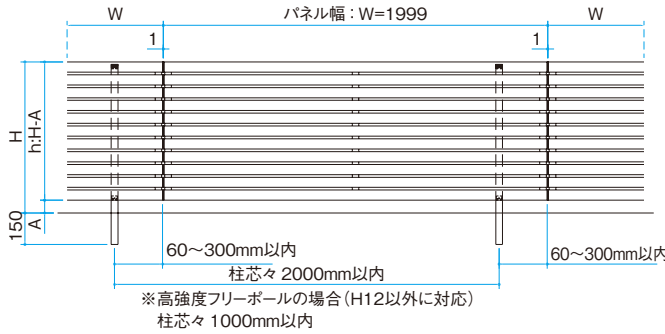
フリーポール仕様時の納まり図
