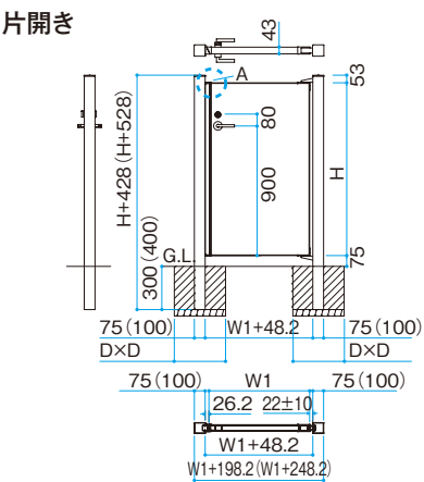
A拡大図
