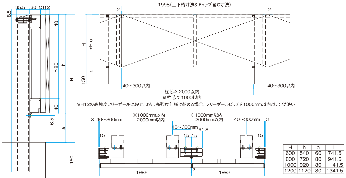
フリーポール 仕様時の納まり図
