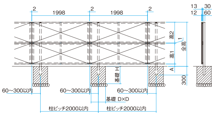
2段フリーポール 仕様時の納まり図
