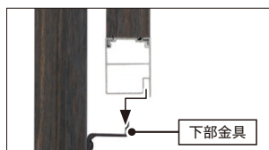
下部金具にフェンス本体をかけます
