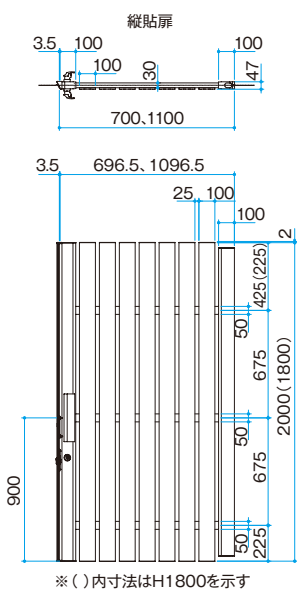
■縦貼扉 別注対応サイズ
