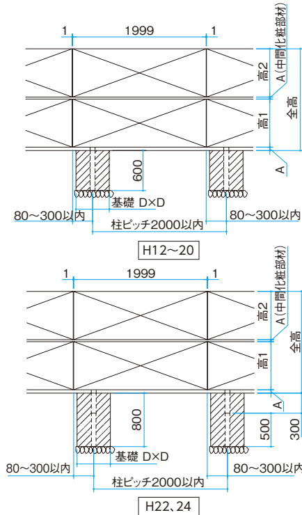
2段フリーポール仕様時の納まり図
