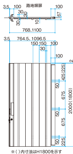
■路地塀扉 別注対応サイズ
