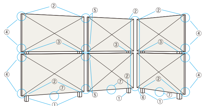
【2段フリーポール納まりの拾い出し例】
