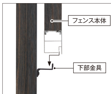
下部金具にフェンス本体をかけます
