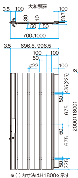
■大和塀扉 別注対応サイズ
